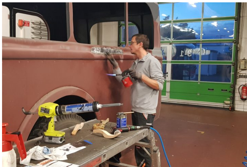
Andreas Fest verzinkt Unebenheiten im Blech des Busses. (Foto: Kraftverkehr e.V.)
